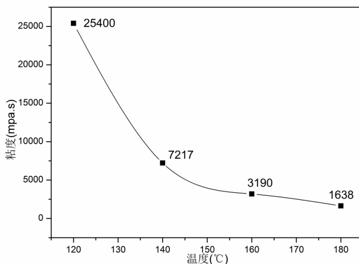
图1、热熔胶粘度随温度变化曲线图
